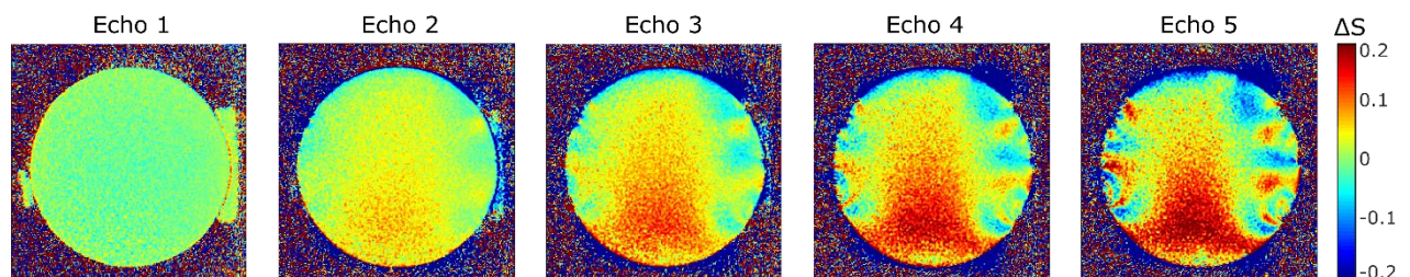
Abb. 1: Signalunterschiede \Delta S , die zwischen den fünf Echos der SE und ME Aufnahmen (Auflösung = (0.75 \text{ mm})^3 , TR = 33 \text{ ms} , FA = 10^\circ , T_{RO} = 1 \text{ ms} , Projektionen = 10000) bestimmt wurden, dargestellt für eine beispielhafte, koronale Schicht.
