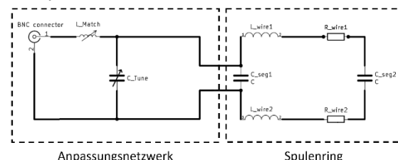
Abbildung 1: Schaltungsdiagramm einer 2-fach segmentierten Spule.
