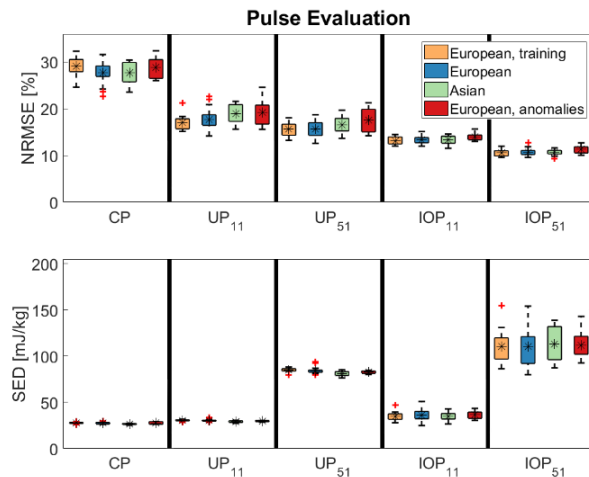
Abb. 2: NRMSE- und SED-Werte aller Pulse für alle Gruppen. Sämtliche UP zeigen niedrigere NRMSE-Werte für alle Gruppen als CP-Pulse. Individuell optimierte Pulse (IOP ij ) zeigen noch bessere NRMSE-Werte und höhere SED-Werte als die zugehörigen UP. IOP 11 zeigt aber sowohl niedrigere NRMSE- als auch SED-Werte als UP 51 .
